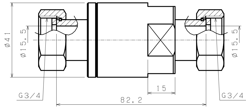
UFB継手RV20 (短) (両ナット)
